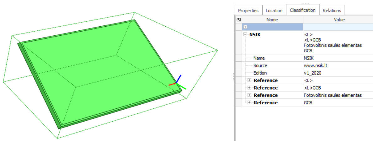
32 pav. Saulės elemento klasifikavimo kodinio žymėjimo perteikimas IfcClassification ir IfcClassificationReference informacinėmis klasėmis
