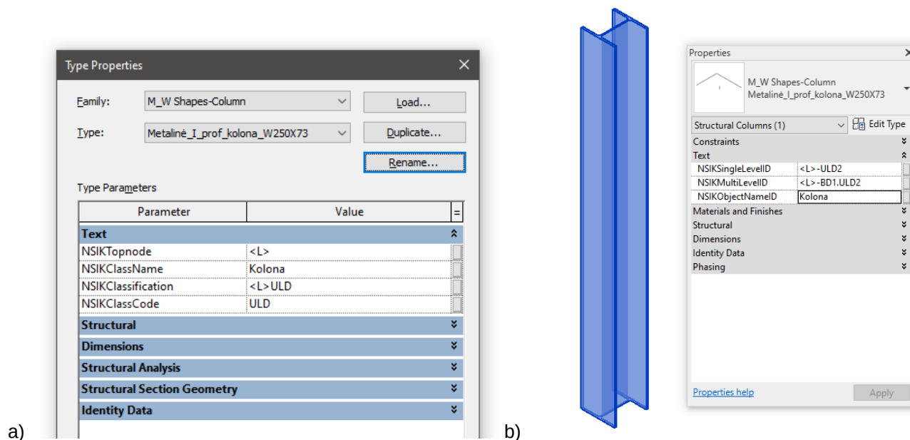
25 pav. Kolonos NSIK kodinis žymėjimas tipiniais (a) ir egzemplioriaus (b) atributais BIM PĮ
