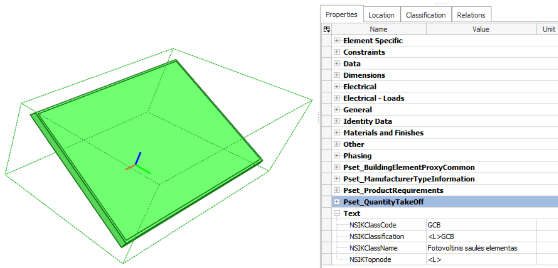
32 pav. Saulės elemento klasifikavimo kodinio žymėjimo perteikimas IfcClassification ir IfcClassificationReference informacinėmis klasėmis
