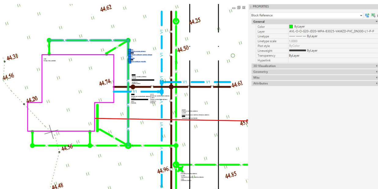
26 pav. NSIK taikymo CAD sluoksnių atributuose pavyzdys
