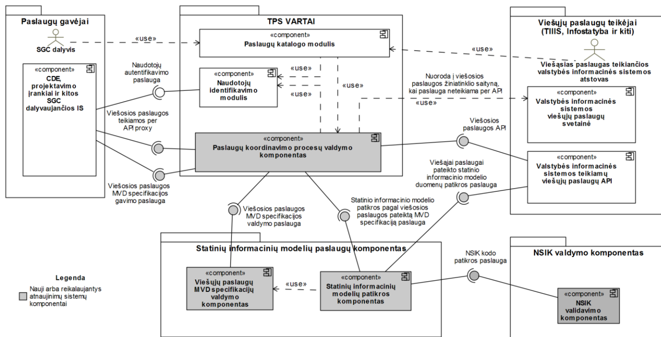
1 pav. Principinė SGC dalyvių ir valstybės informacinių sistemų sąveikumo, apsiikeičiant statinio informaciniais modeliais, architektūra
